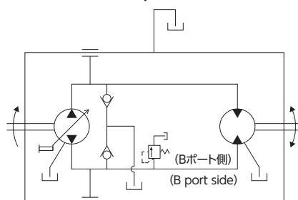
油圧回路図 / Hydraulic circuit
