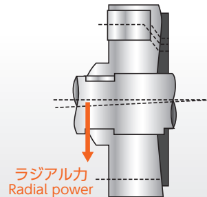
球面バルブプレート図 / SVP design
